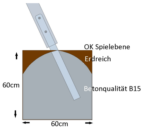
Querschnitt- Fundament A
