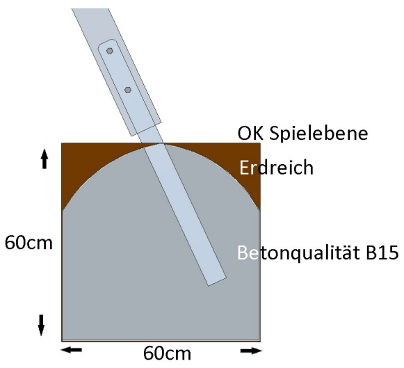
Querschnitt- Fundament A
