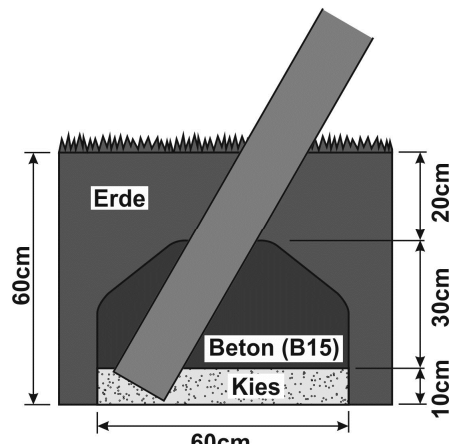
Querschnitt-Fundament A
